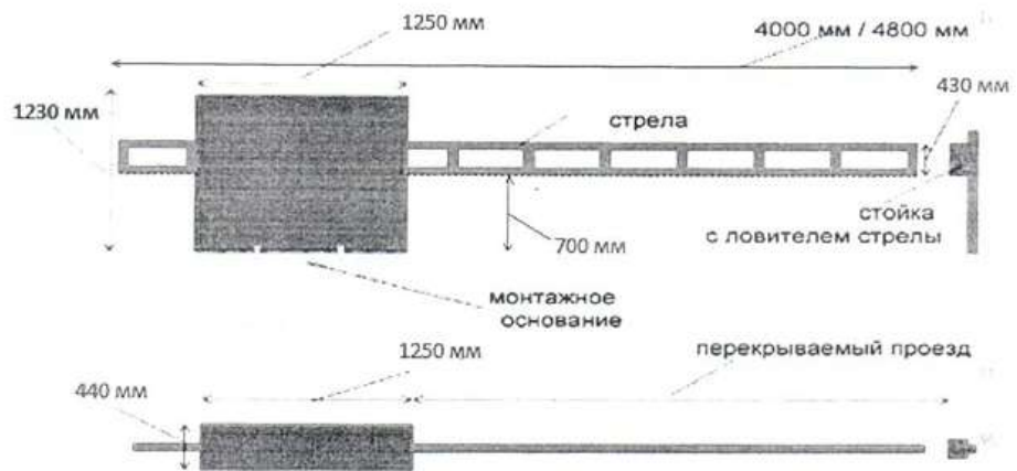
Рис. 2 Размеры шлагбаума
