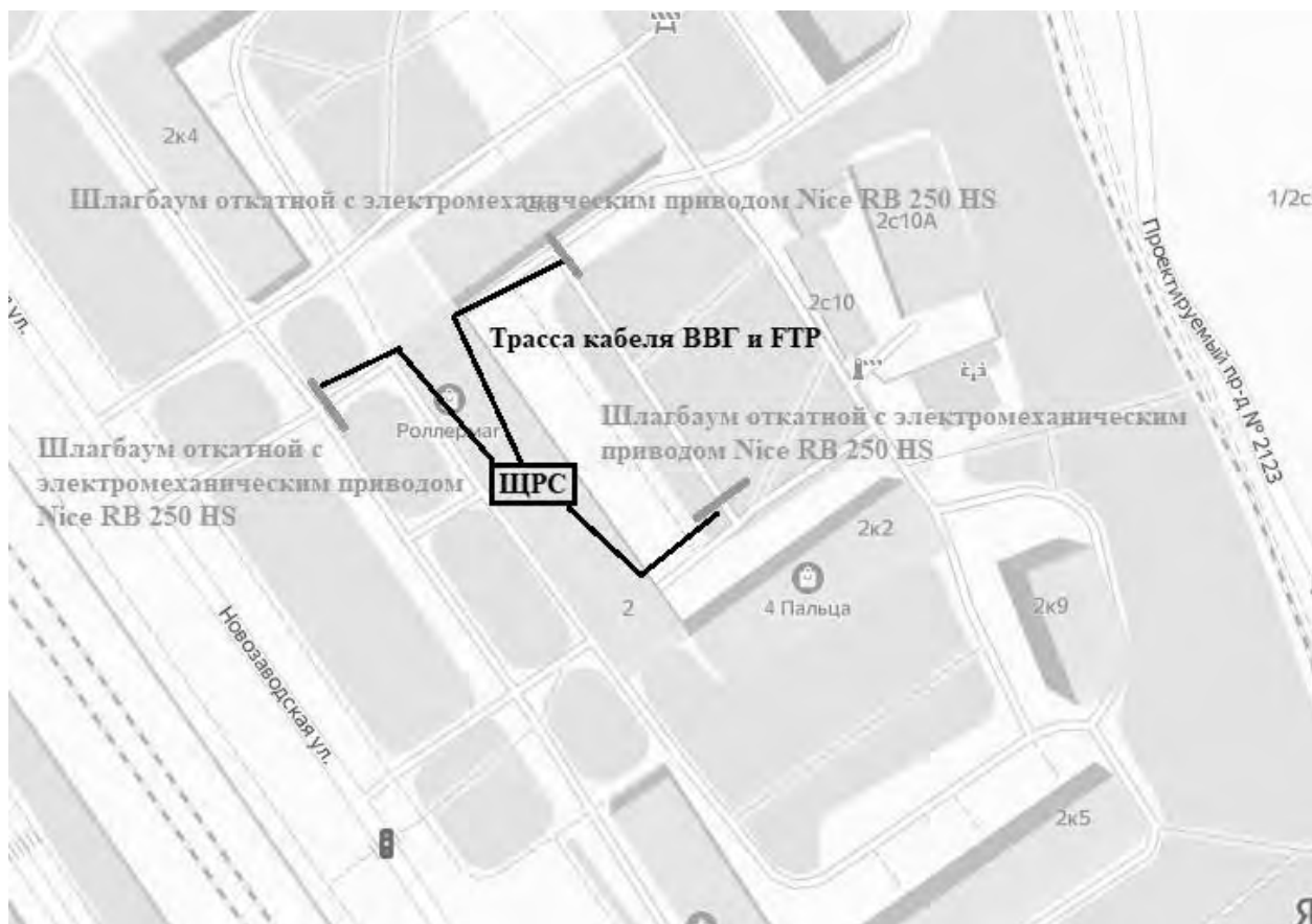
Схема размещения шлагбаумов
