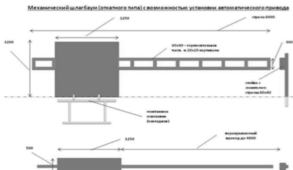
Рис.3. Внешний вид шлагбаума
