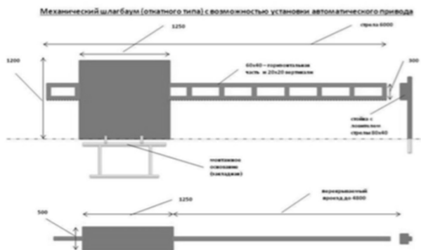
Рис.3. Внешний вид шлагбаума
